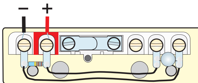
Anslutningsplintar i fotocellen.
