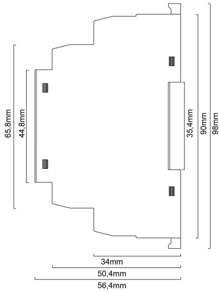
geometry din rail
