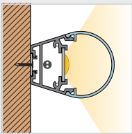
Wandmontage mit Aluminiumträger wall mounting with aluminium carrier
