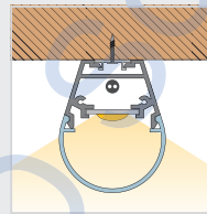
Deckenmontage mit Aluminiumträger ceiling mounting with aluminium carrier
