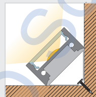
Montage mit Eckhalter mounting with corner bracket
