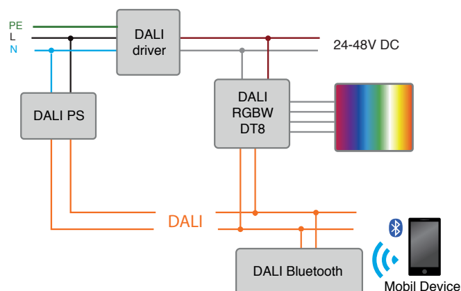
Typisk oppsett for farge- og fargetemperaturstyring:
