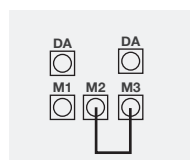
V2: Dimming 10-100% Under 1V: OFF (Rød karakteristikk)
