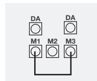
V4: Dimming 10-100% Under 1V: Min (10%) (Blå karakteristikk)
