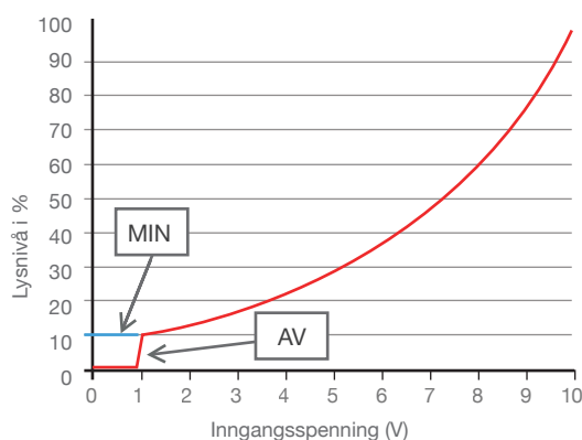
Lysnivå på en DALI driver med 0/1-10V inngang
